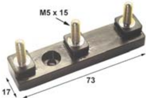
REF 107TA1629 For fuse: DIN 72581/72582 Used for: JUNGHEINRICH
