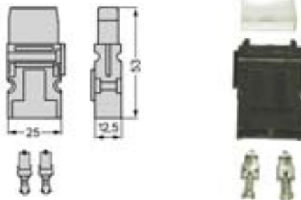
REF 106TA2730 For fuse: DIN 72581 / MED
