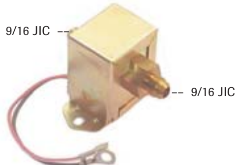
REF 115TA1808 24 V
