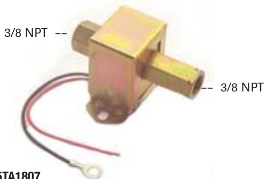
REF 115TA1807 24 V
